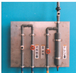
給気・排気、マスフロメーター 取り付けパネル
